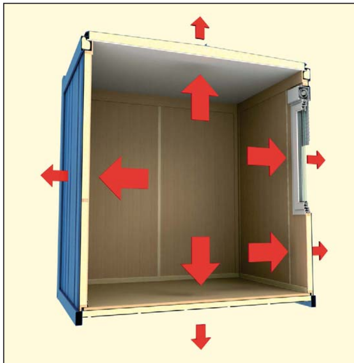
Isolierungen im Schnitt
